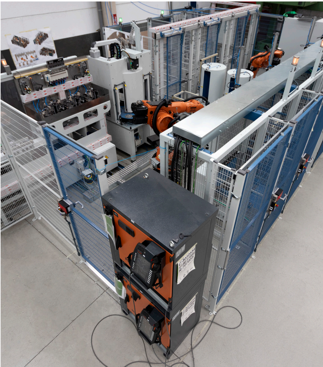
Almacén automatizado de herramientas
