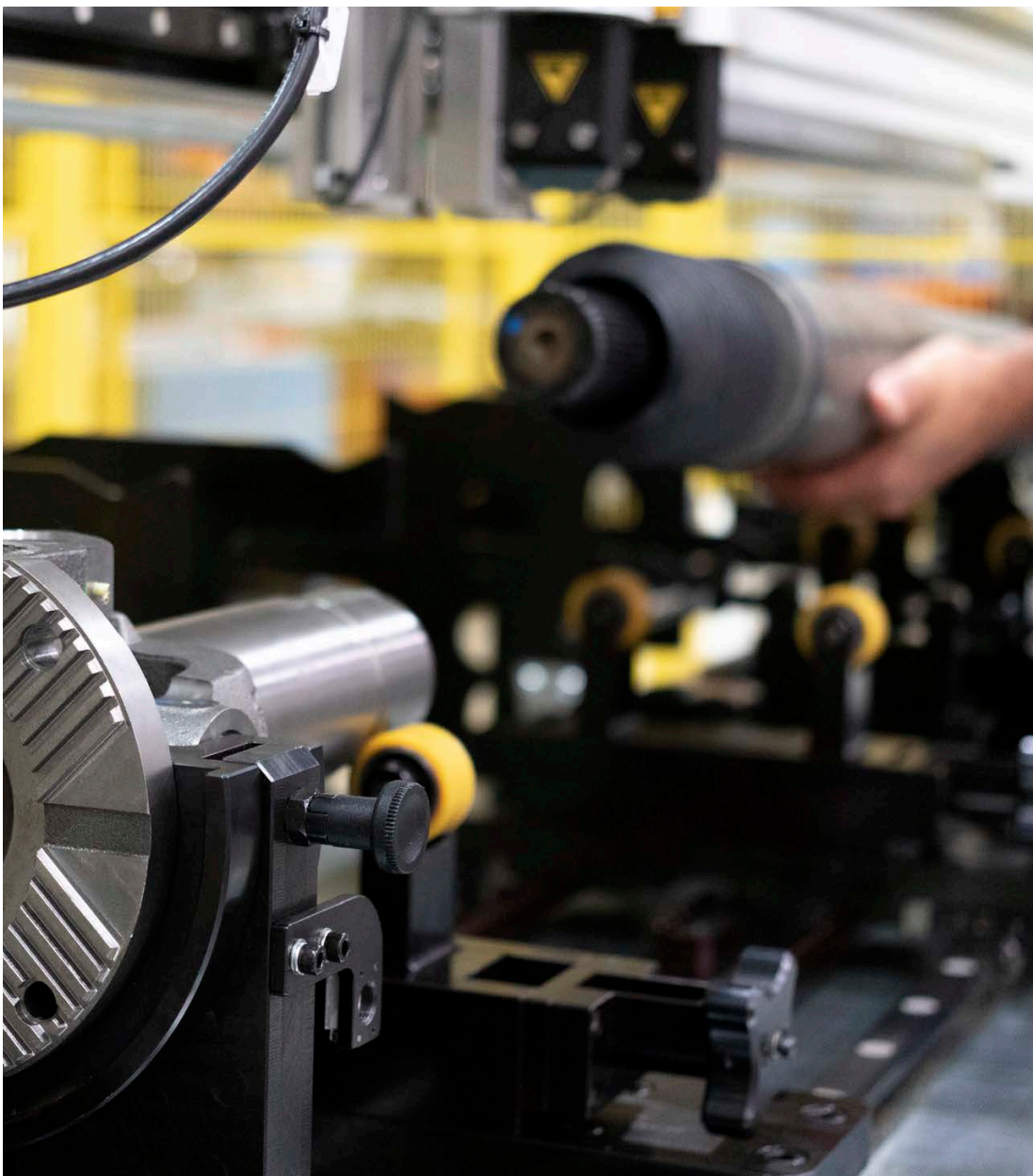
Máquina montaje de propshafts
